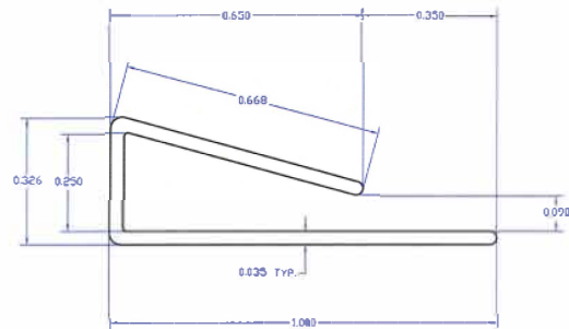
Edge J-Trim
