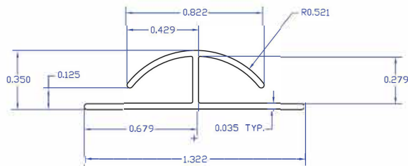
Divider Trim
